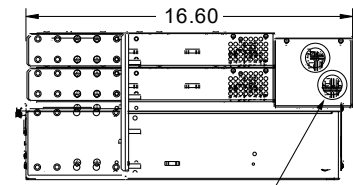
Right Side View Diam. 1.38 (2-places)
